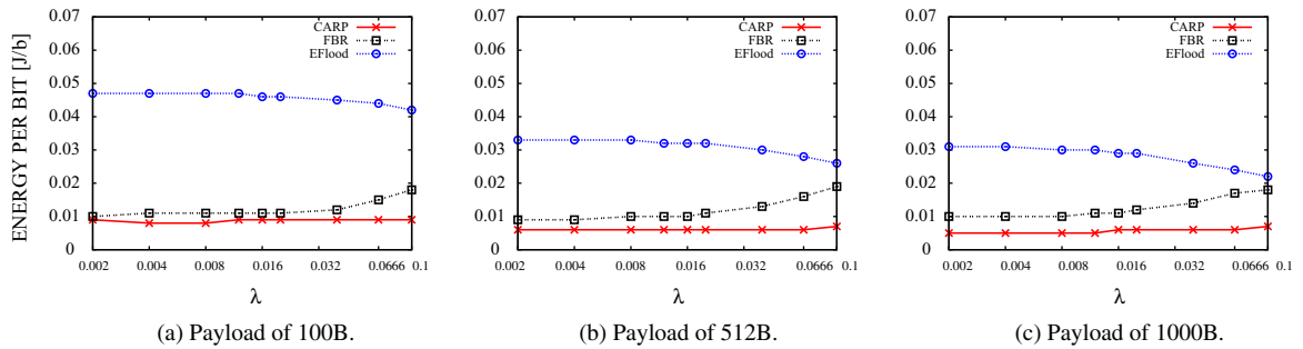
Fig. 3. Energy per bit.
